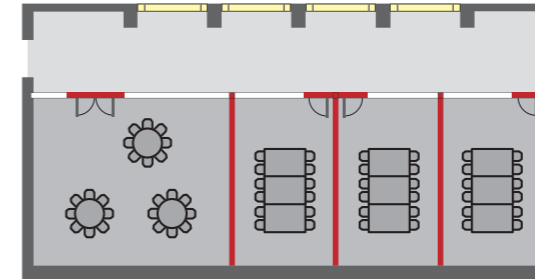
Situace, kdy místnosti navazují na chodbu (chodba propojující místnosti)
