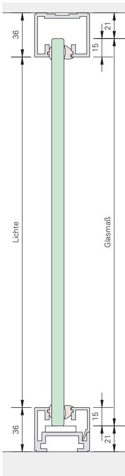
MR 36 kombiniert mit MR 36 U bei grossen Massdifferenzen
