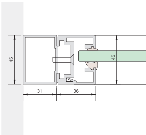
MR 36 Rahmen mit Zusatzprofil 31/45 zum Ausgleich bei bauseitigen Sockelleisten
