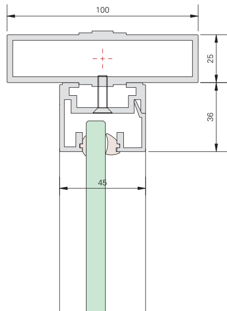
Waagrecht Abschlussprofil für freistehende Elemente ohne Deckenanbindung
