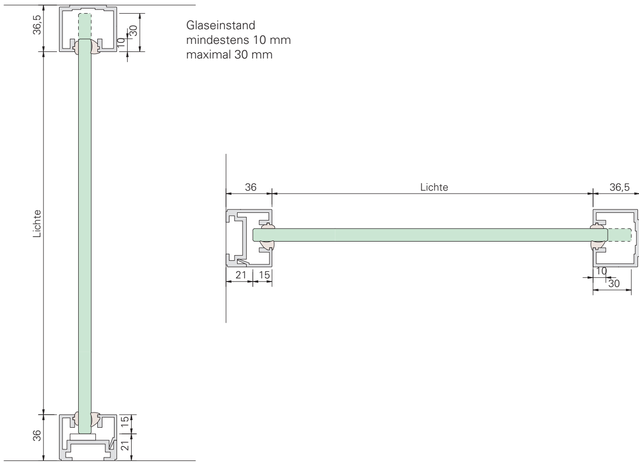
MR 36 kombiniert mit MRU 36 bei großen Maßdifferenzen (wird auf Stoß ohne Eckverbinder verarbeitet)
