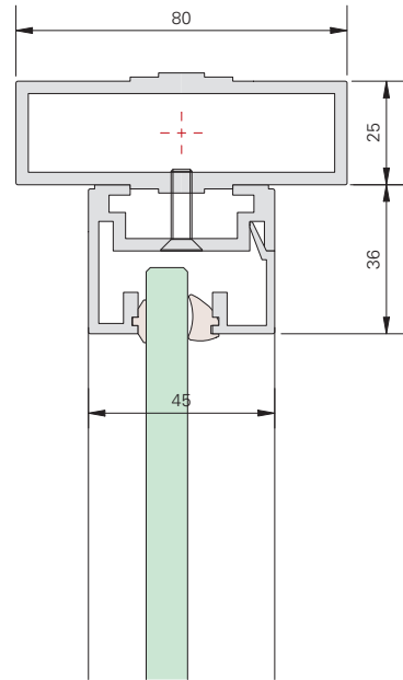
Waagrecht Abschlussprofil für freistehende Elemente ohne Deckenanbindung
