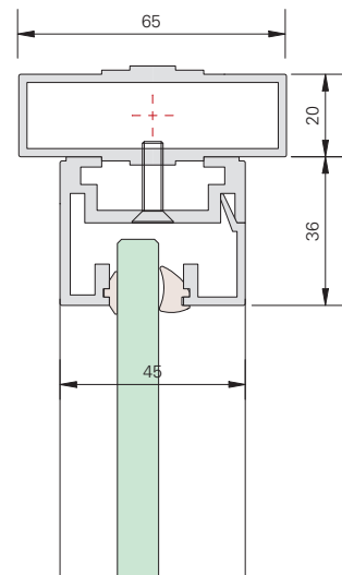
Waagrechtes Abschlussprofil für freistehende Elemente ohne Deckenanbindung
