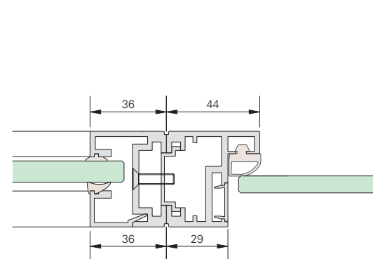
MR 36 Rahmen und AT 44 Anschlagtürzarge mit Easy-Connection
