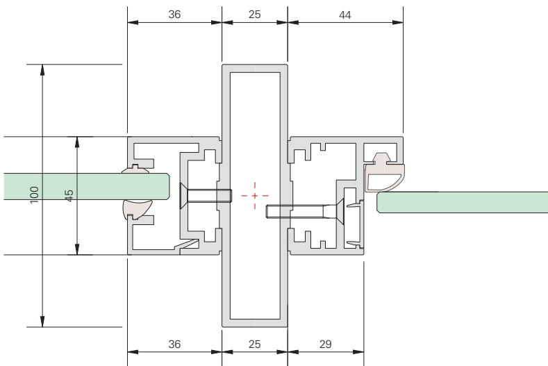
Senkrecht Stabilisierungsprofil für hohe Elemente für MR 36 Rahmen und AT 44 Anschlagtürzarge
