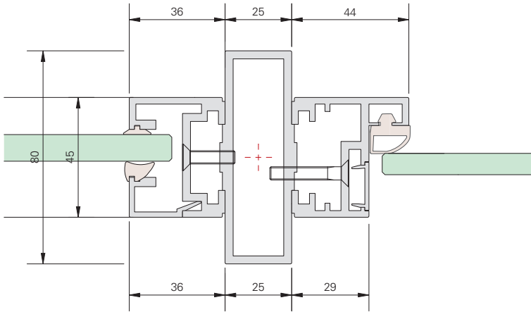
Senkrecht Stabilisierungsprofil für hohe Elemente für MR 36 Rahmen und AT 44 Anschlagtürzarge
